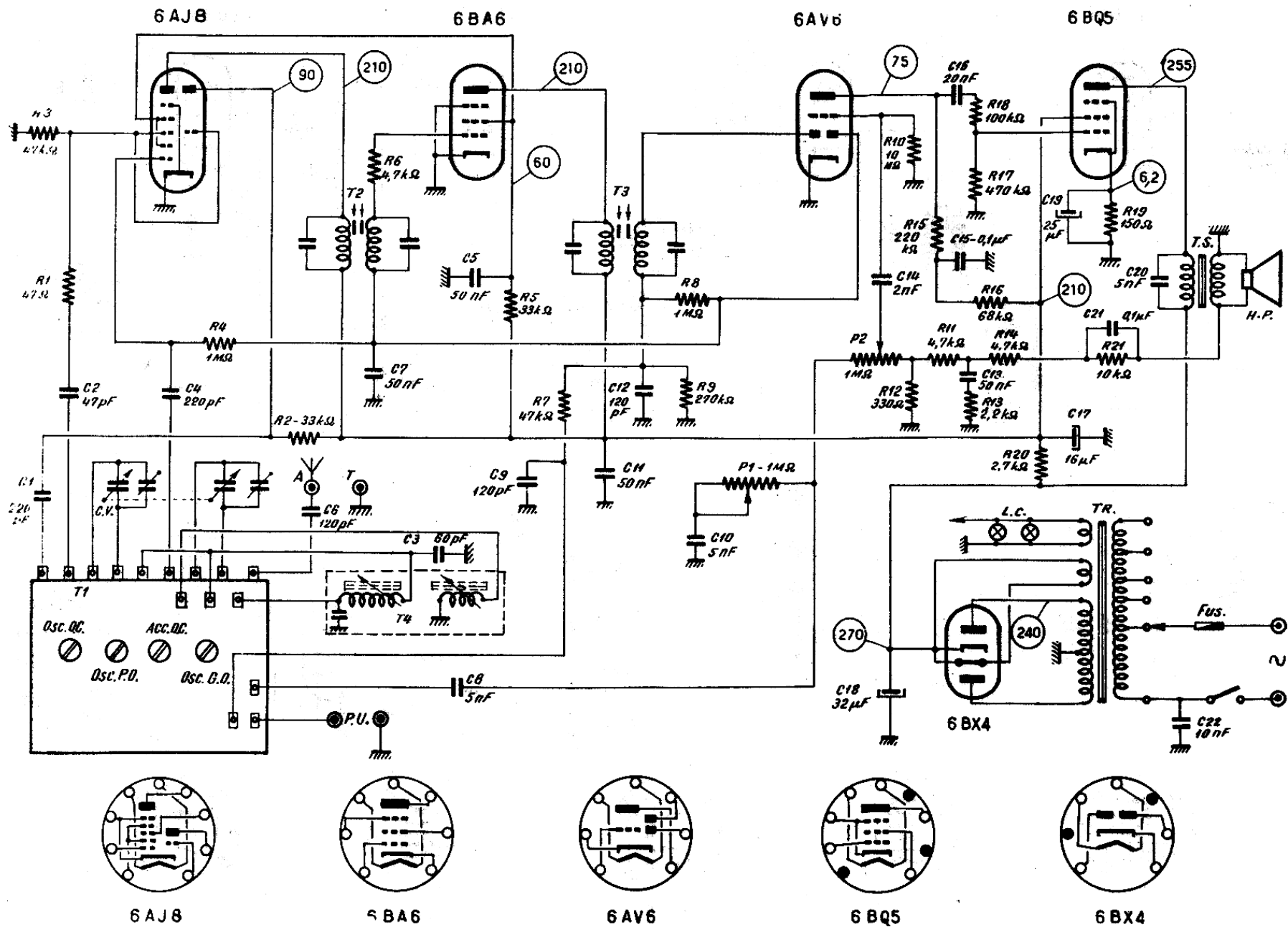
Schéma général du récepteur 5715.
